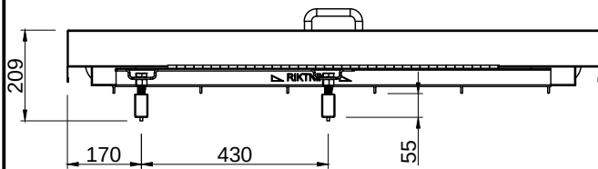
Front aanzicht
